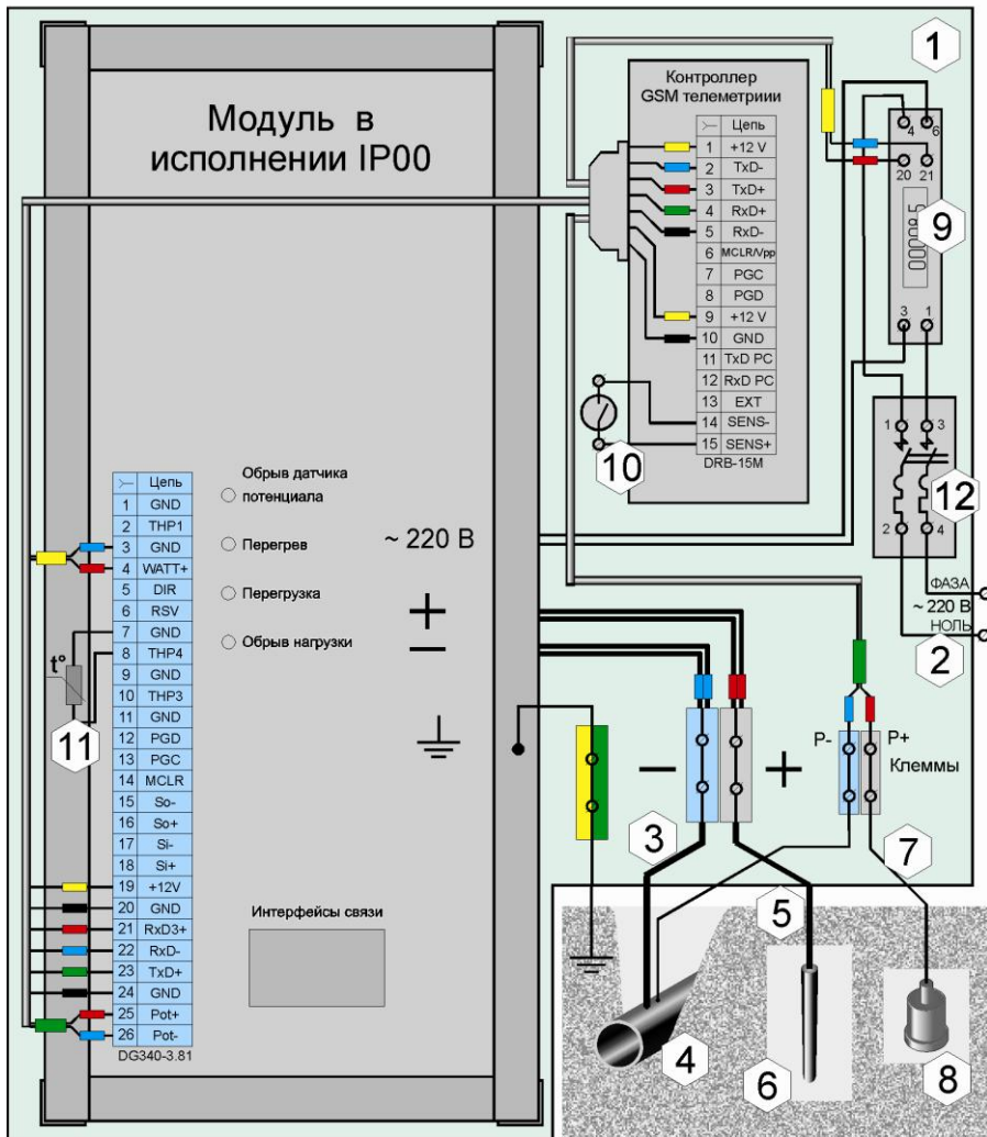
Схема электрическая устройства типа "ТИЭЛЛА" на основе одного модуля
